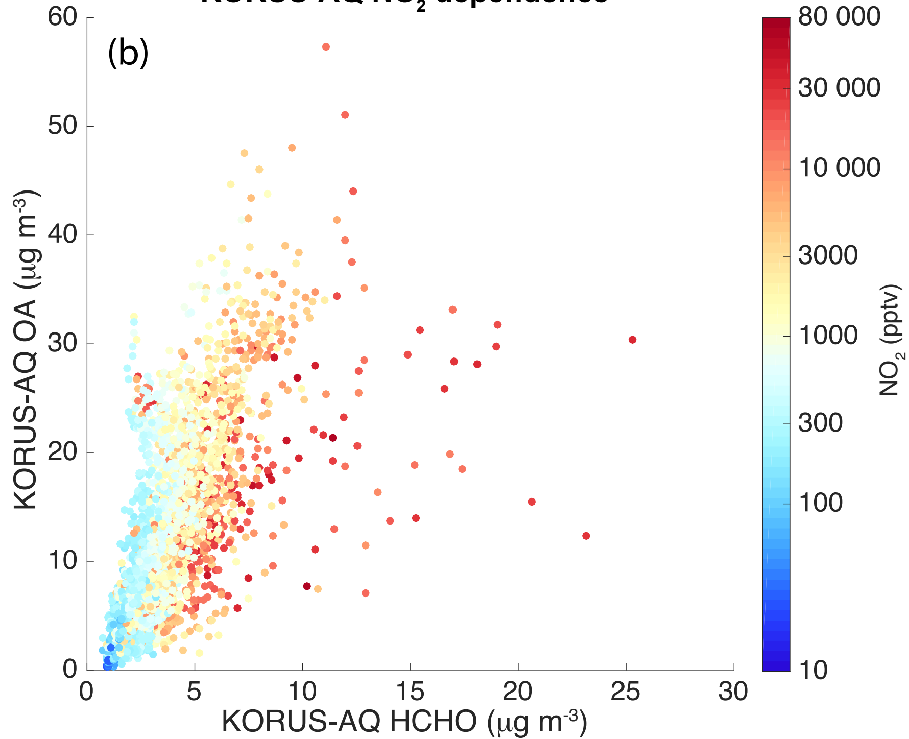
KORUS-AQ NO 2 dependence
