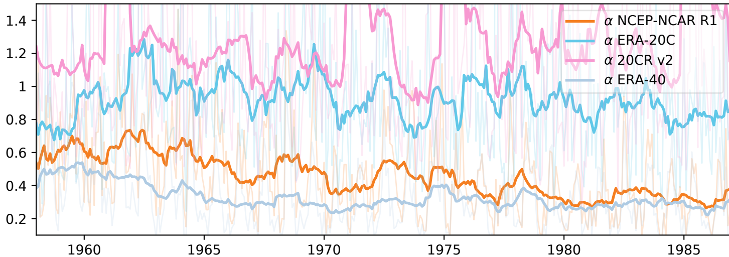
(b) u 500 hPa 45° S
