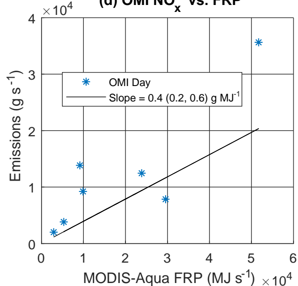
(d) OMI NO x vs. FRP
