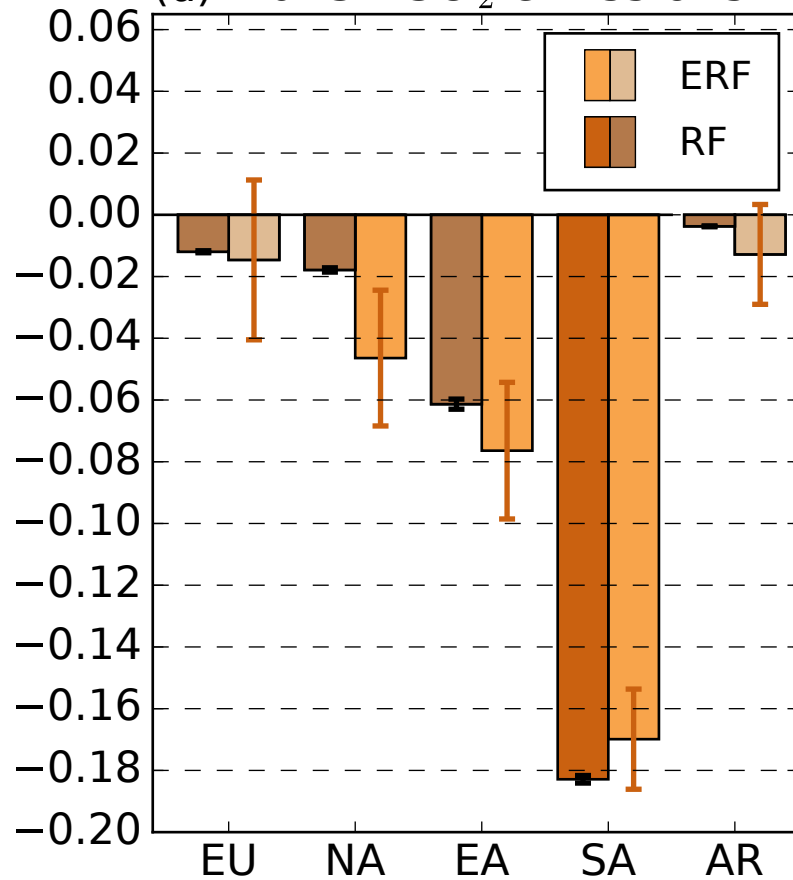
(d) 10xSA SO 2 emissions
