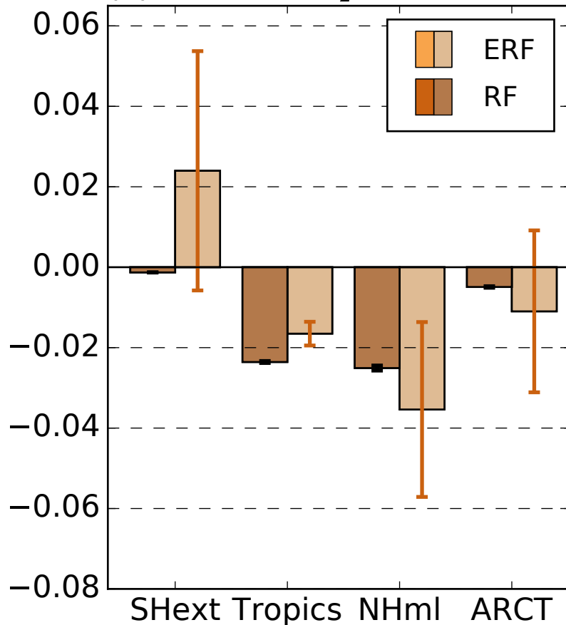
(d) 10xSA SO 2 emissions
