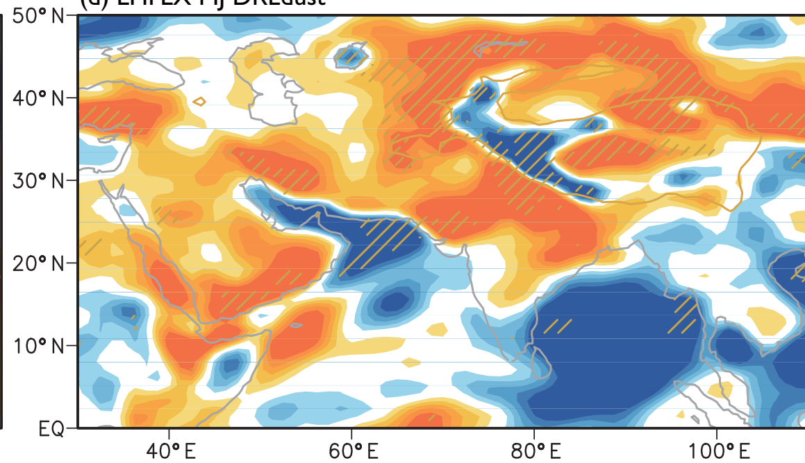
(d) LHFLX MJ DREdust
