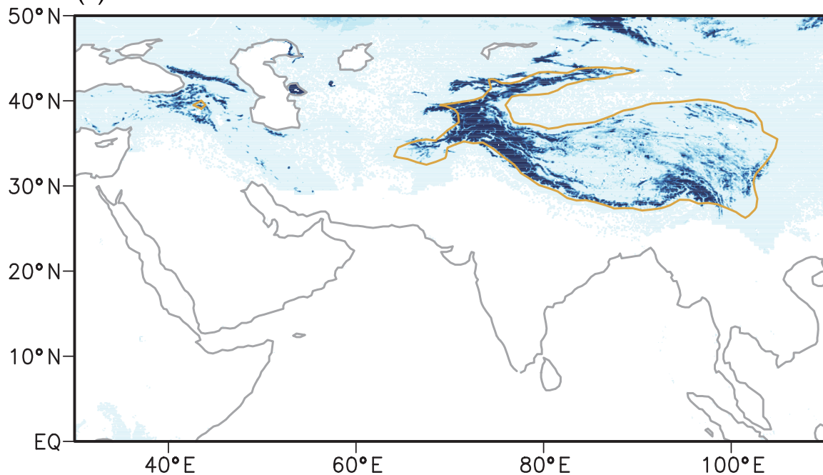
(d) MODIS snow cover fraction APR
