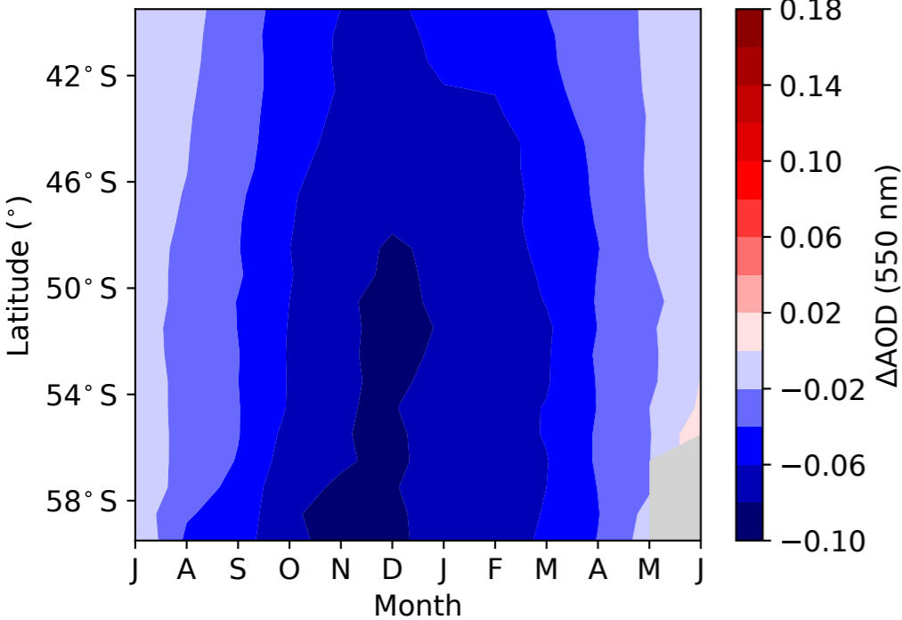
(d) CHEM1-SSF minus MODIS [RMSE=0.052]
