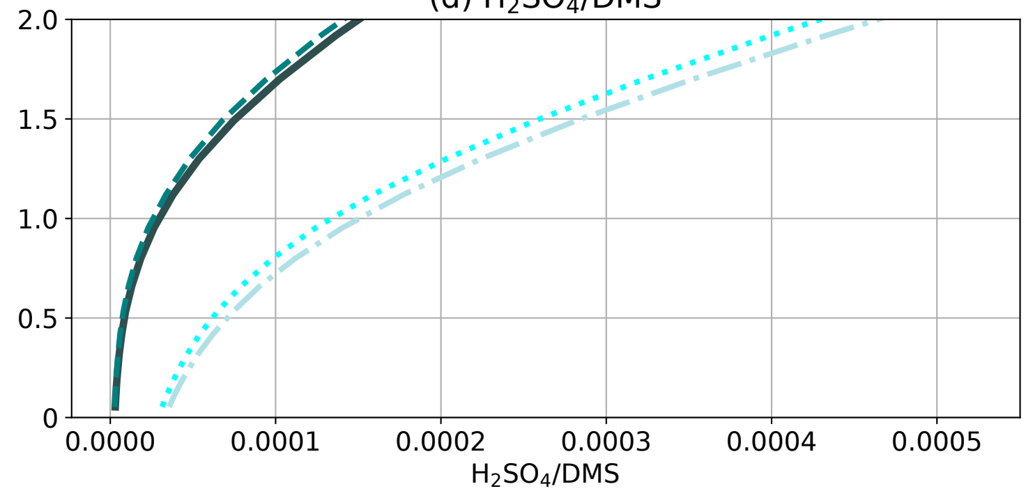
(d) H 2 SO 4 /DMS
