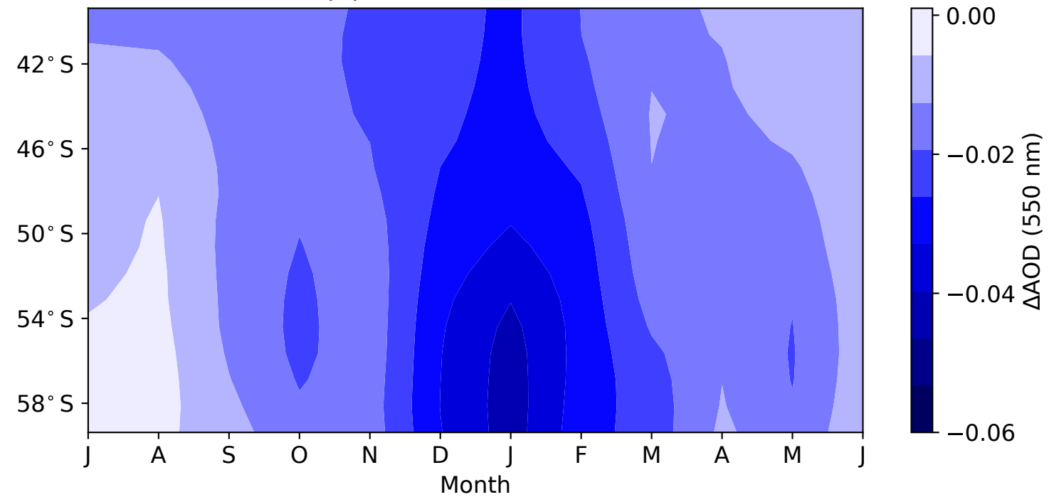
(d) NODMS minus REF
