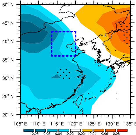
(d) SON SLP reg. onto AHD_{BTH}
