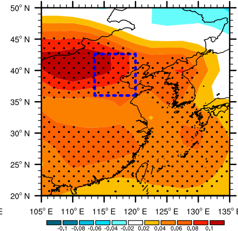
(b) SON Ts reg. onto AHD_{BTH}
