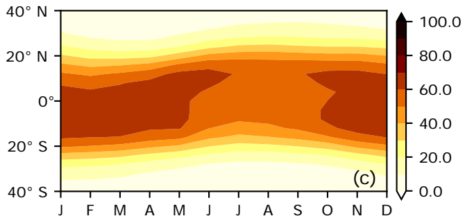
RH
