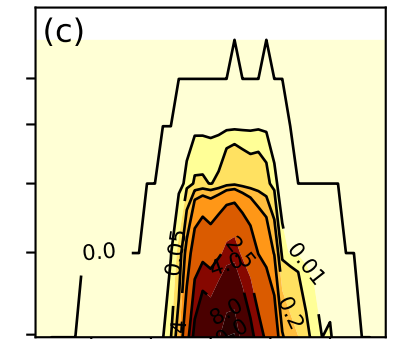
GEOSCCM
