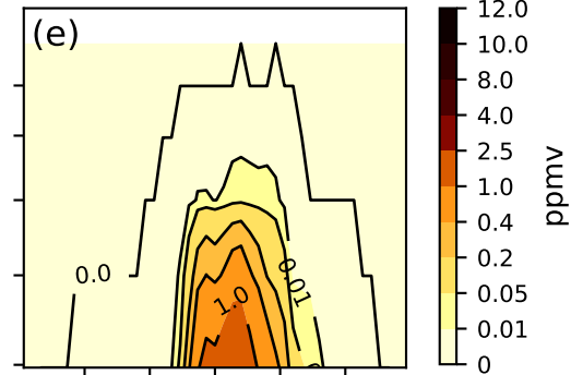
GEOSCCM 0.2ice
