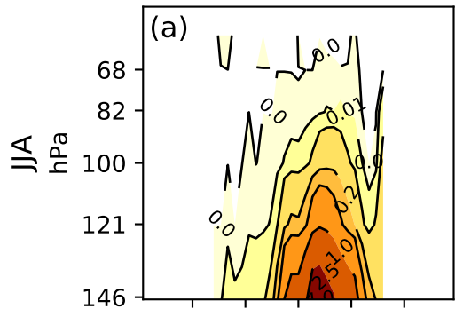
CALIOP
