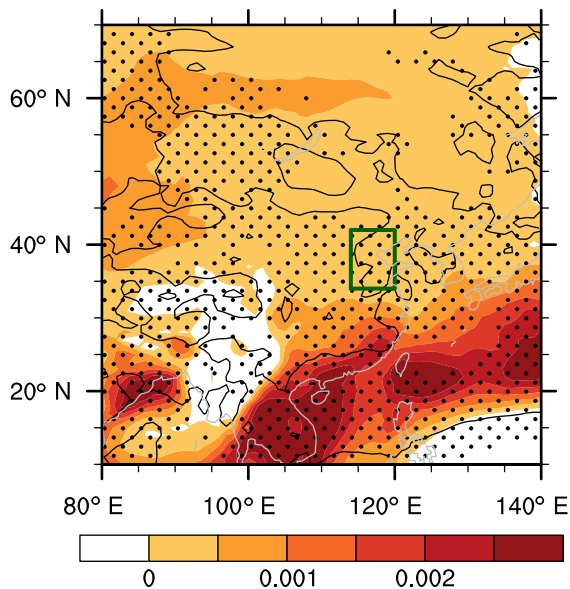
(d) Shum, BLH, WSPD
