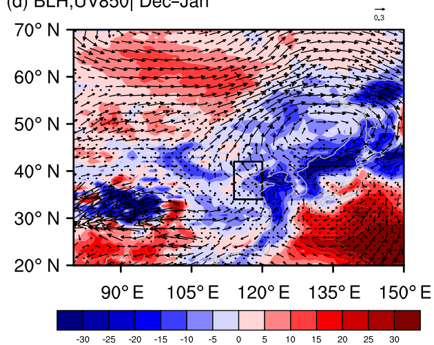
(d) BLH,UV850| Dec-Jan
