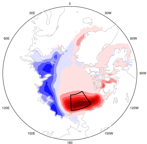
(a) SI| Sep-Oct
