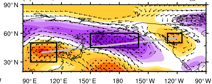
(d) SLP,UV
