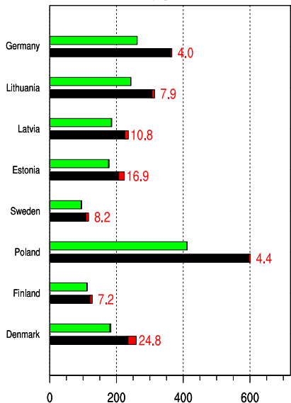
(d) Dep. oxidised sulphur in mgS m -2
