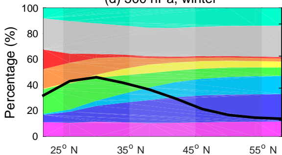
(d) 500 hPa, winter
