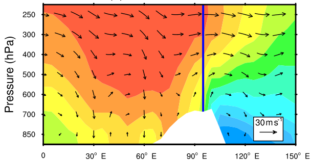
(d) Winter, 20–40° N
