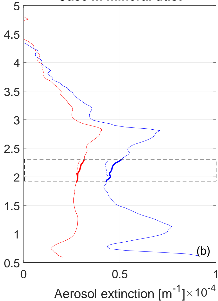
Case II: mineral dust
