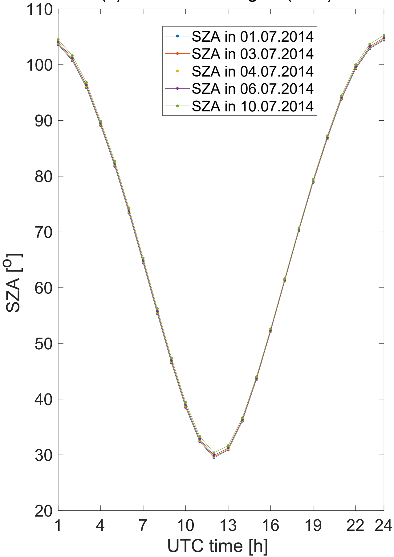
(a) Solar zenith angles (SZA)
