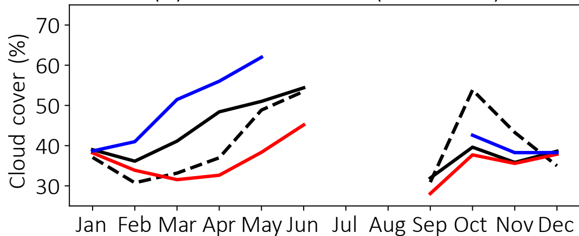
(d) Snow covered (liquid clouds)
