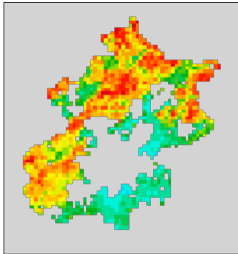
(b) MODIS: JJA
