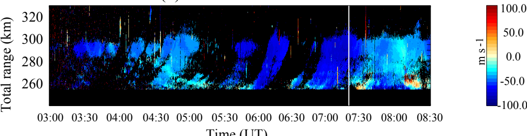
(d) Horizontal wind
