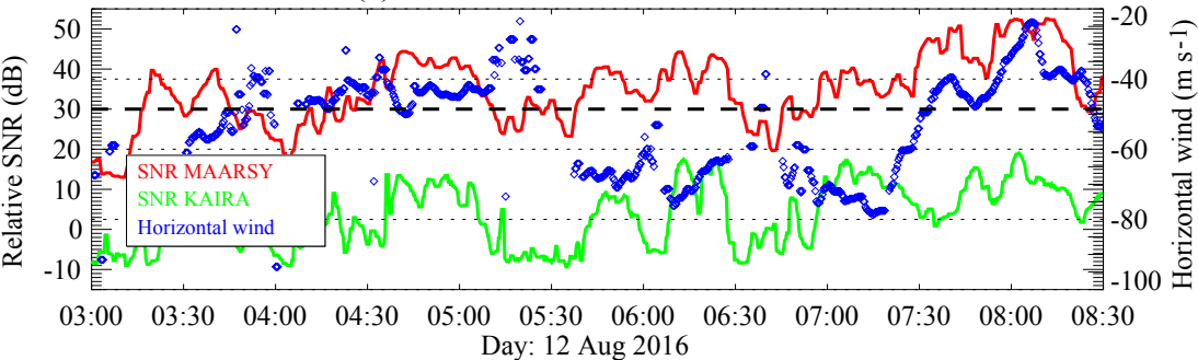
(a) PMSE SNR over MAARSY
