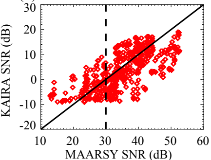
(b) SNR MAARSY vs. KAIRA
