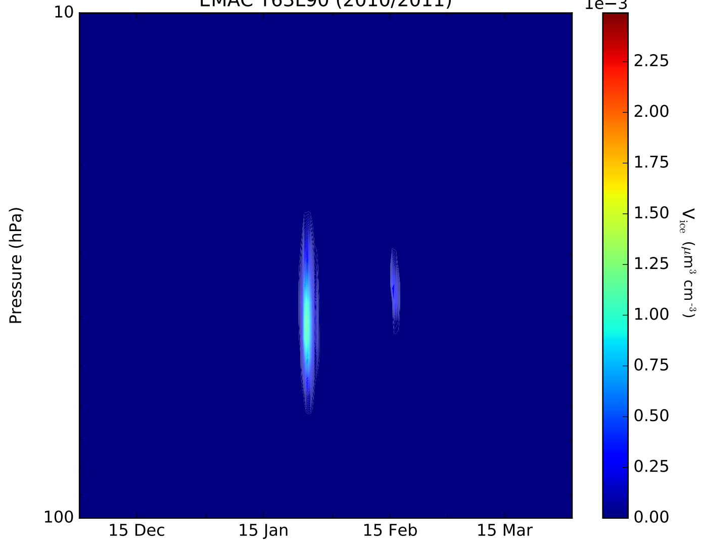
EMAC T63L90 (2010/2011)
