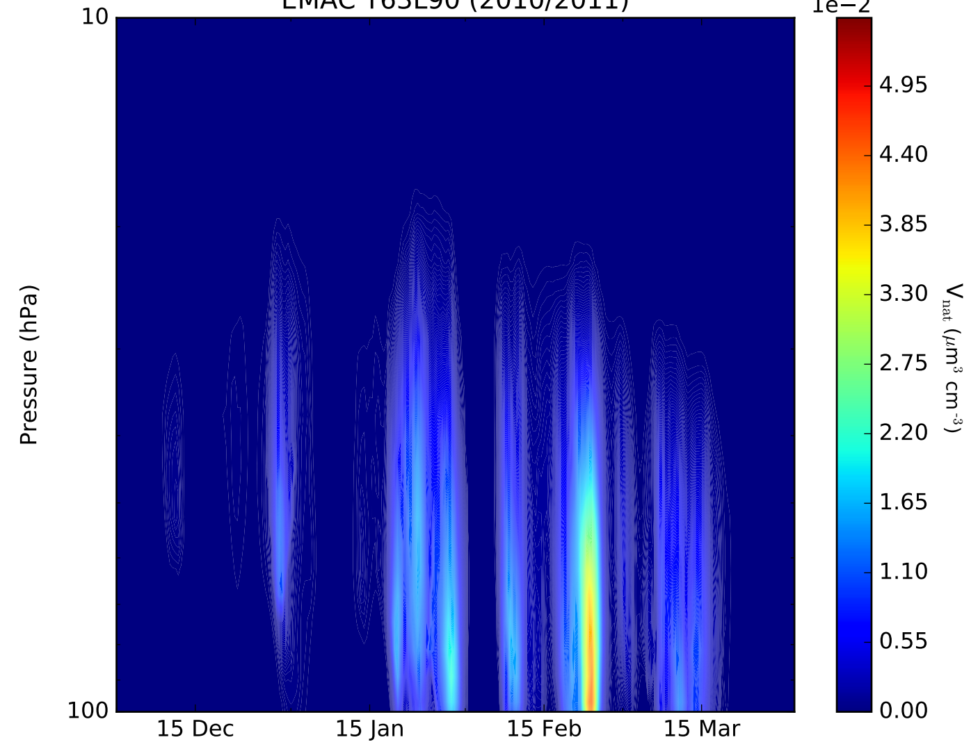
EMAC T63L90 (2010/2011)
