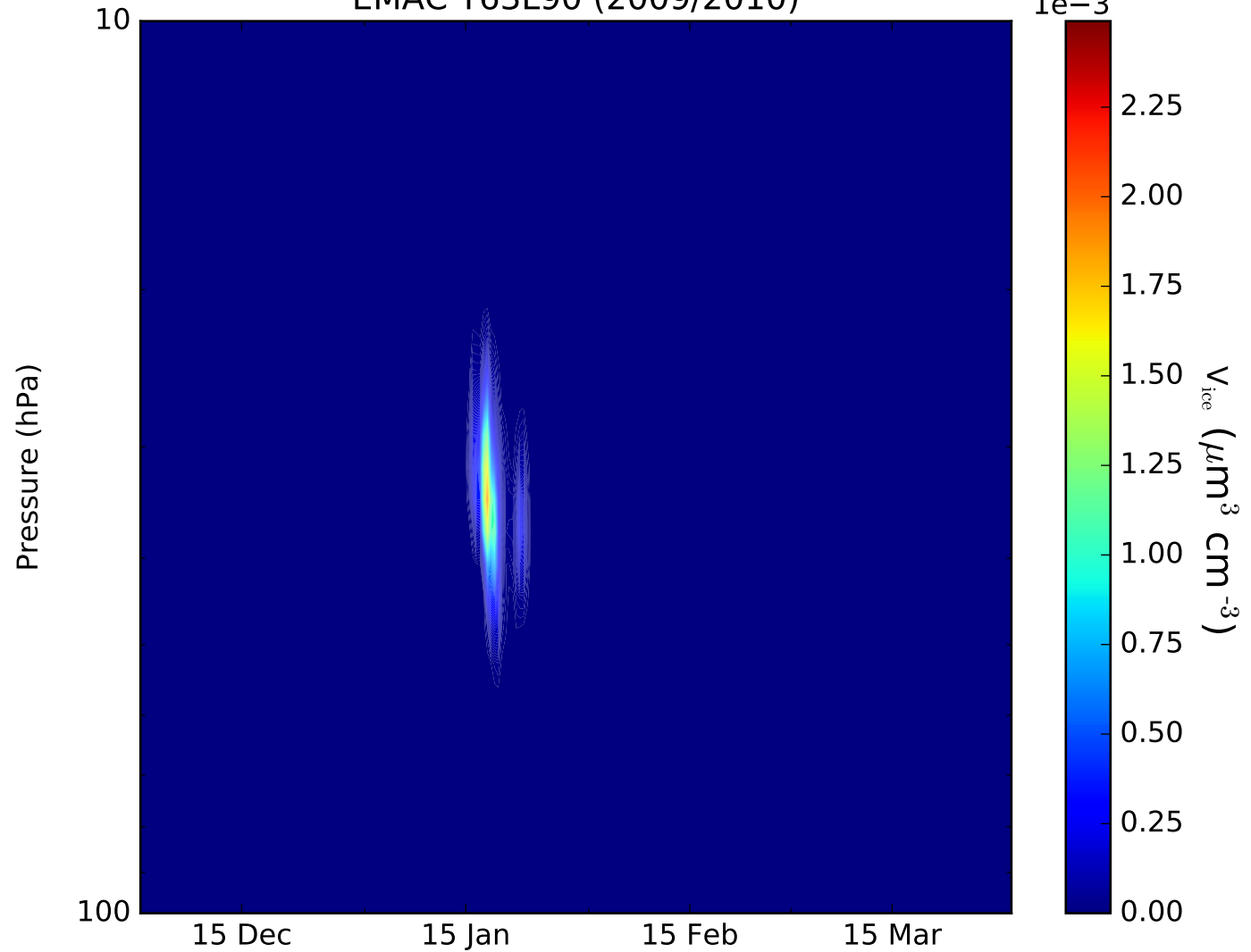
EMAC T63L90 (2009/2010)
