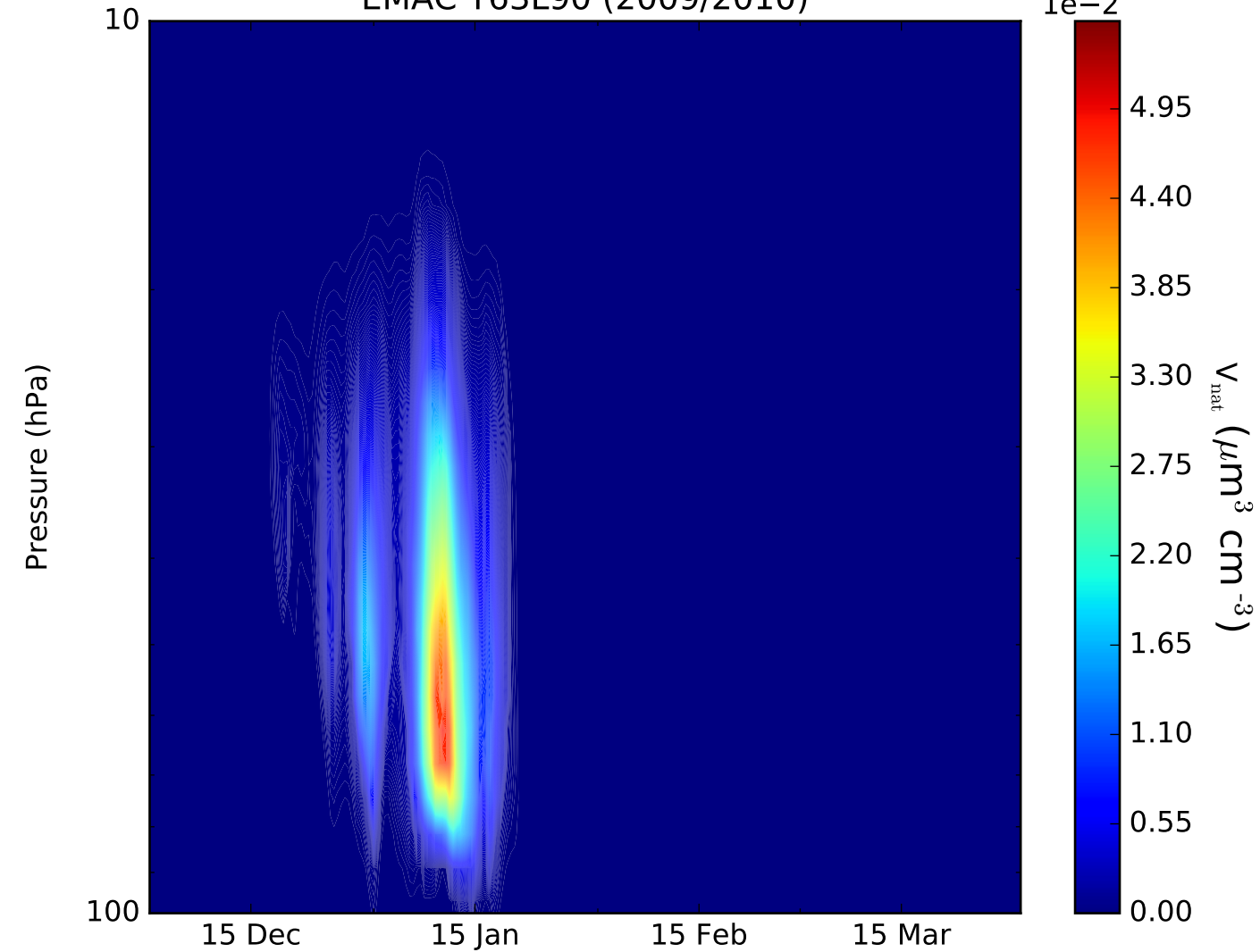
EMAC T63L90 (2009/2010)
