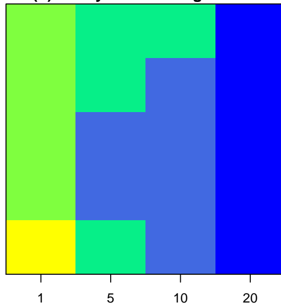
(d) Rocky Mountains grid cell
