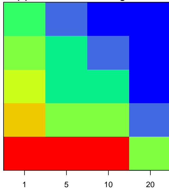
(d) Rocky Mountains grid cell
