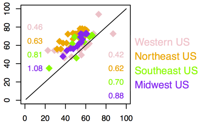
(d) Present-day CAM-Chem variability [%]
