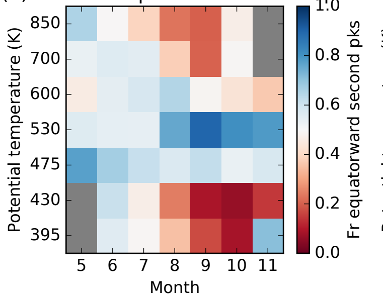
(d) Fraction equatorward second peaks
