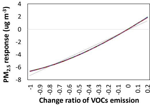
(d) VOCs
