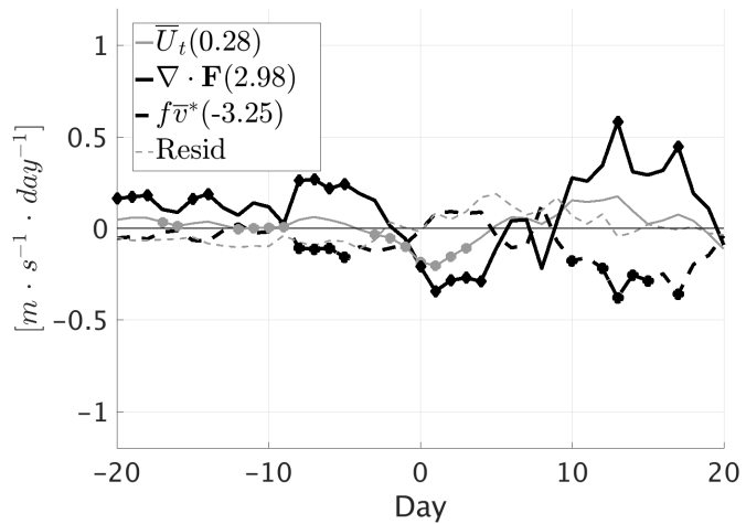
(d) Momentum budget ( \frac{m}{s \cdot day} ), 50–0.1 hPa, WQBO
