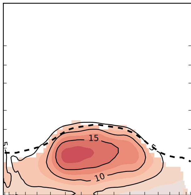
(b) Lightning (Ltn-CIm)
