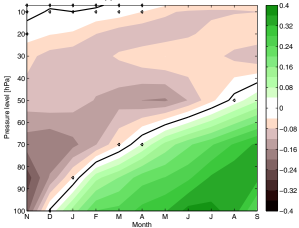
(a) El Nino in 1997/1998
