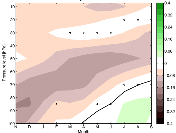
(b) EP El Nino, excluding 1997/1998 and 1982/1983
