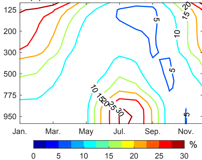
(d) Fractional contribution of SHAF
