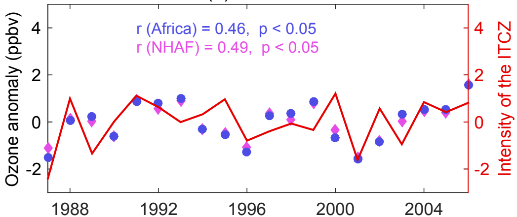
(b) 600 hPa
