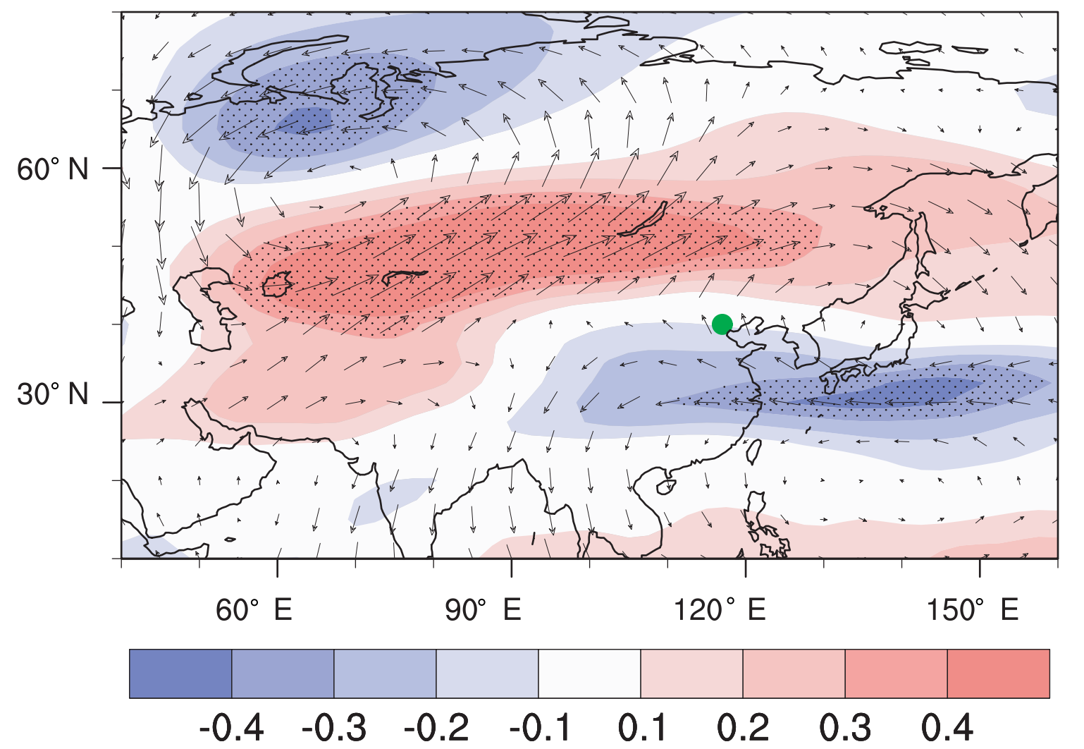
(d) Zonal wind speed and wind at 200 hPa
