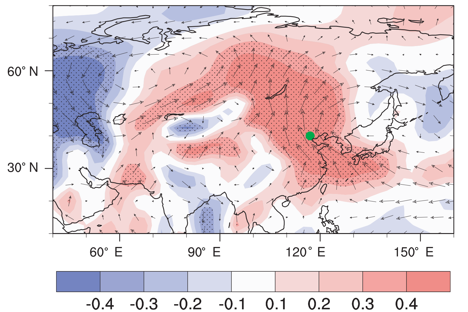
(d) Zonal wind speed and wind at 200 hPa
