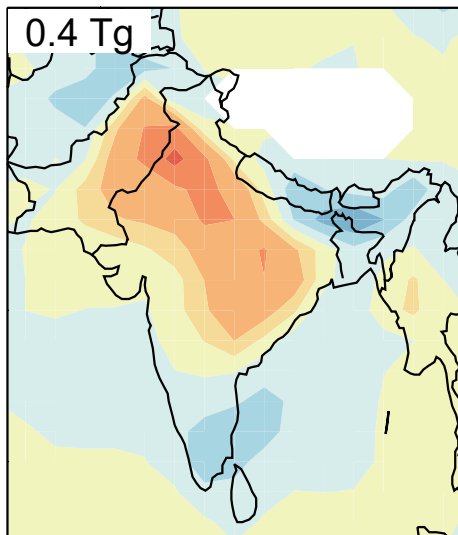
(d) \text{O}_3 net production [ 10^{-3} \text{ kg m}^{-2} ]
