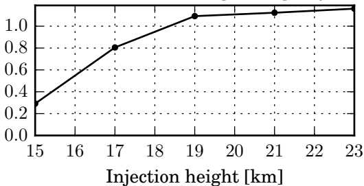
(d) Burden/emission [ \text{Tg(S)} / \text{Tg(S) yr}^{-1} ]
