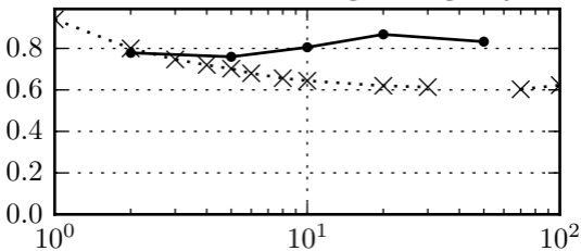
(d) Burden/emission [ \text{Tg(S)} / \text{Tg(S) yr}^{-1} ]
