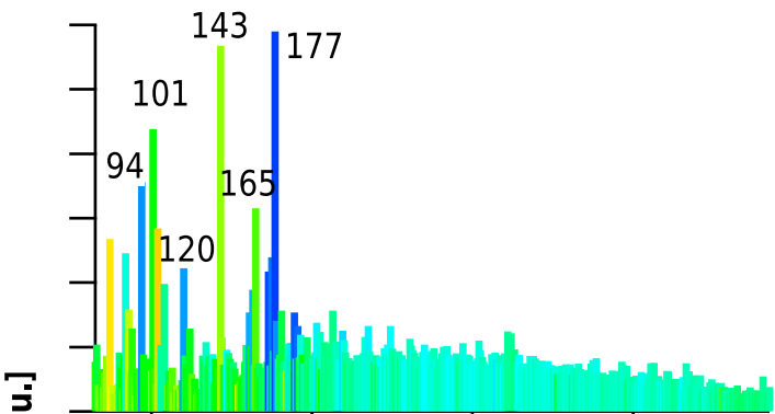
(a) Bern, 2013-08-20, R_{m/z,NOx} summer
