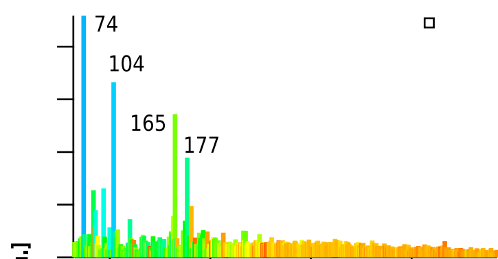
(b) Payerne, 2013-08-20, R_{m/z,temp}
