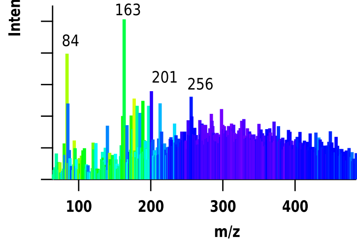
(d) Zurich, 2013-12-14, R_{m/z,levoglucosan}
