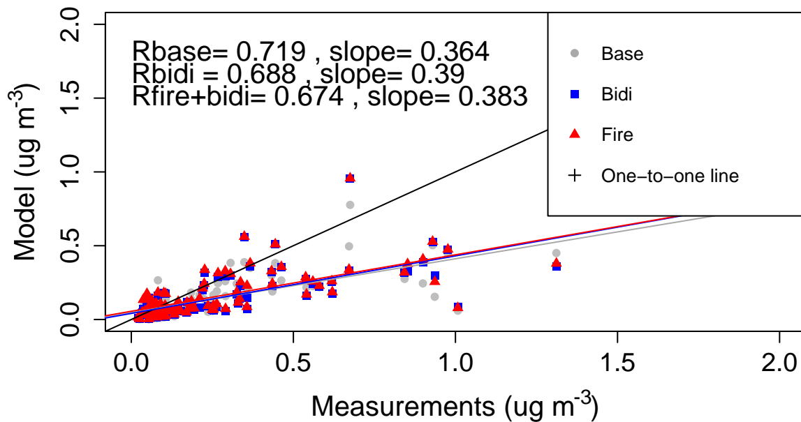
(d) Hourly average NH 4 concentrations on all flight paths
