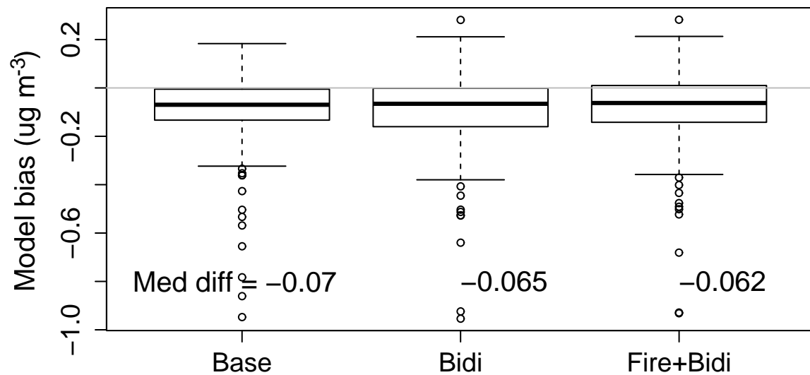
(d) Hourly average NH 4 concentrations on all flight paths
