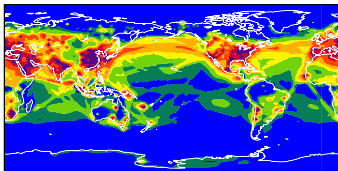
(d) Total sulfate
