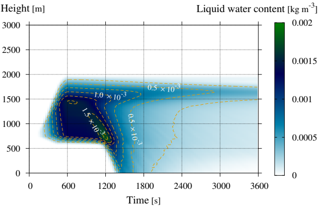
(a) LCS
