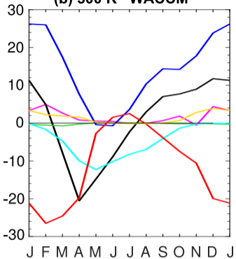
(b) 500 K WACCM
