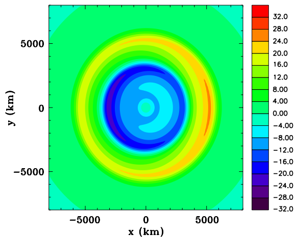
(d) Vertically summed total energy
