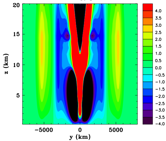
(d) Vertically summed total energy
