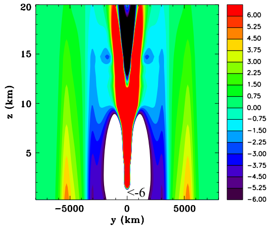
(d) Density perturbation
