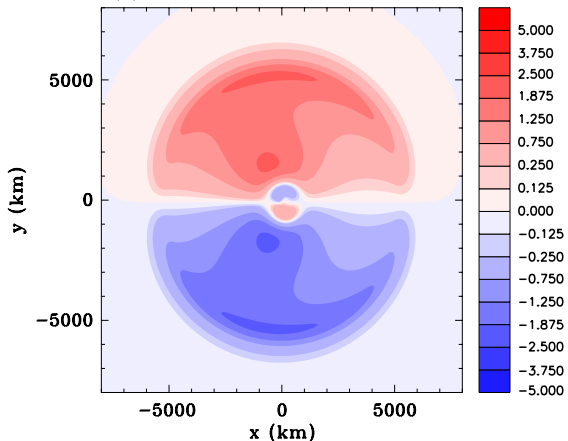
(d) Mass flux
