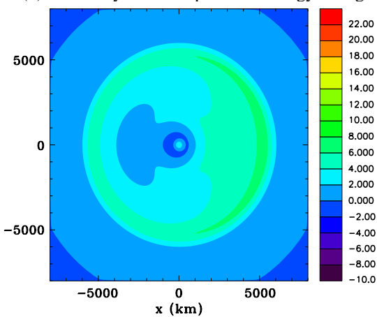
(d) Vertically summed potential energy change
