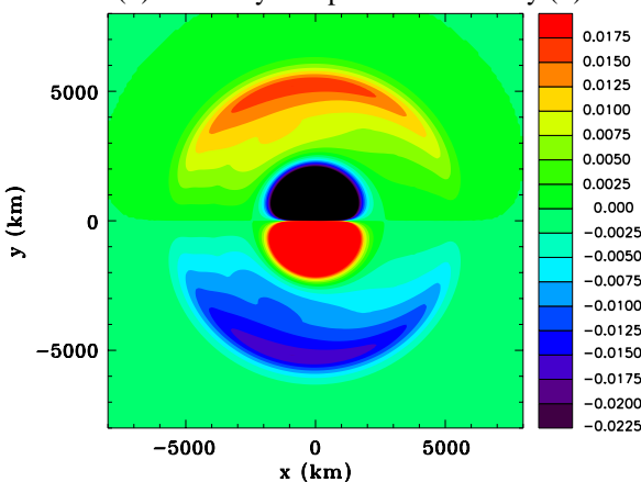
(d) Surface y component of velocity ( v )
